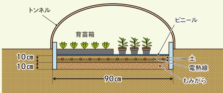
図1 電熱温床
